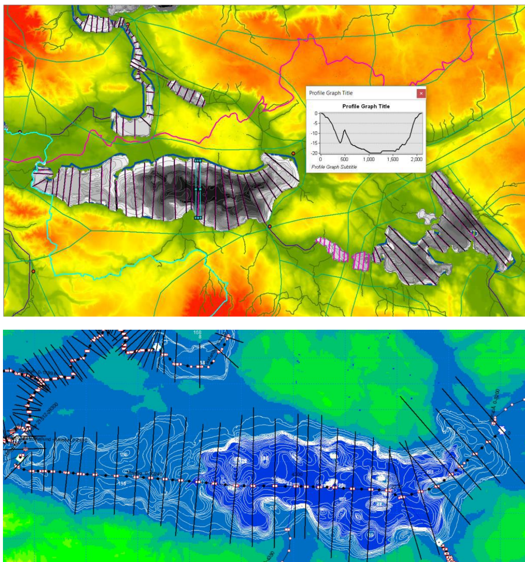
Figur 4-3 Eksempel på tværsnitsdata hentet fra sødybdekort ved Mossø og i vandløbsmodellen efter forlængelse af sø- og vandløbstværnsnit med terrænmodel data. Figuren viser terrænkoter, sødybdekurver, vandløbsnetværk og tværnsnit.
